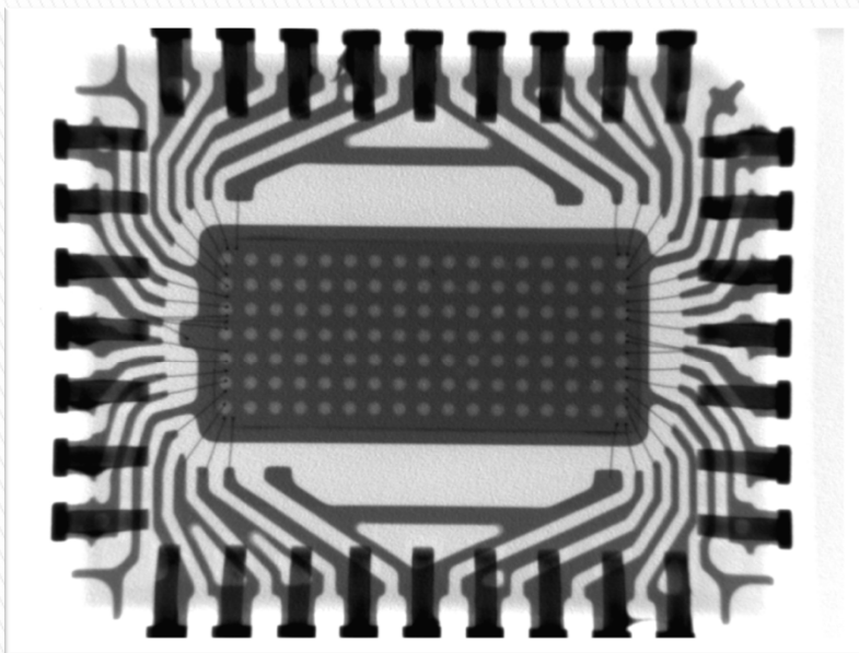
Исправная подделка, 0922(0545), рентген. фото
