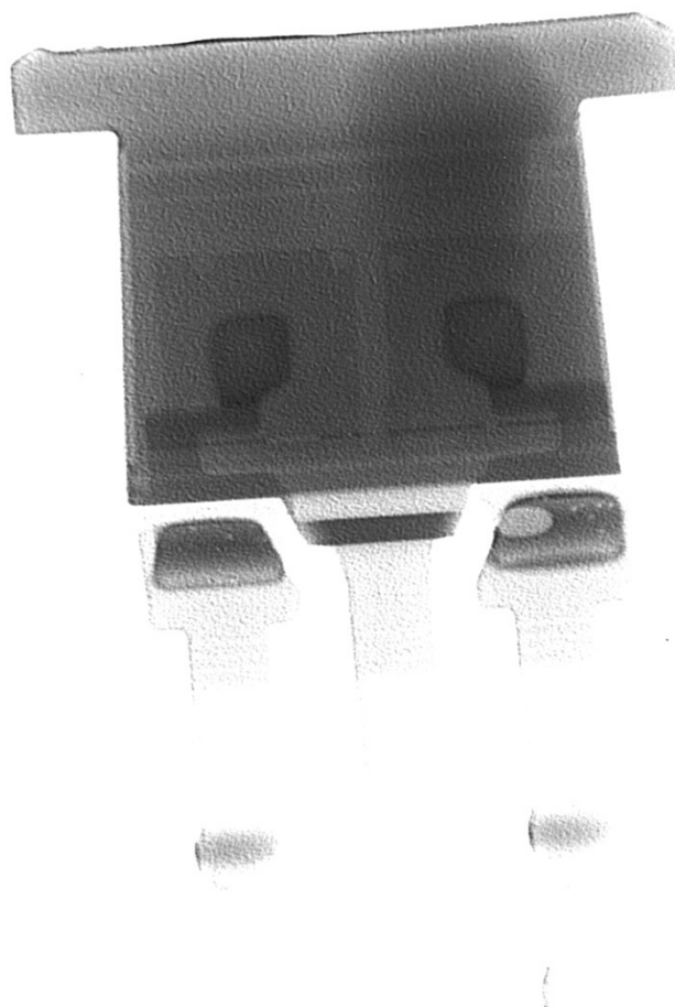
216, рентген. фото, подделка
