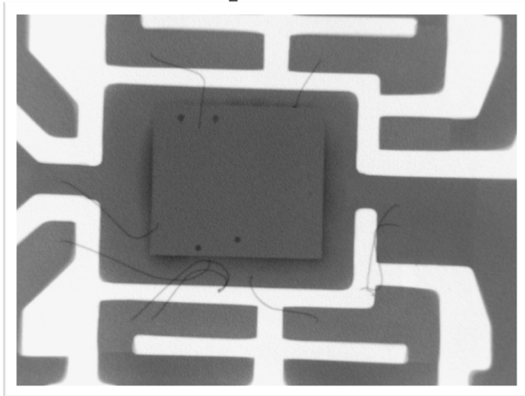
Все выводы в обрыве
