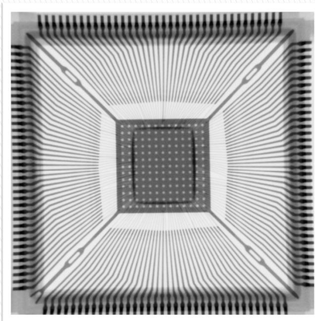
1205, оригинал, рентген. фото
