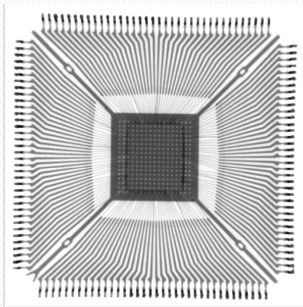
1035, 1043 подделки, рентген. фото
