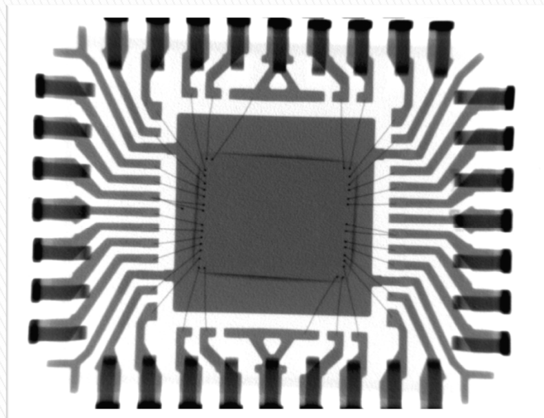
Полная подделка, 0428, рентген. фото
