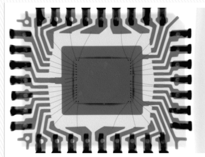
Полная подделка, 0428, рентген. фото
